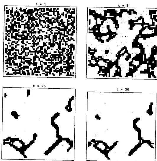
Fig. 9b. k=5 , h=8
