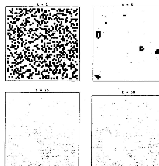
Fig. 9a. k=5 , b=8
