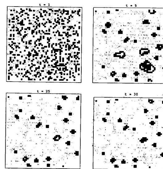
Fig. 11a. k=4 , h=7
