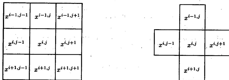
Fig. 15. Intorni ad 8 e 5 celle su un reticolo regolare bidimensionale quadrato
