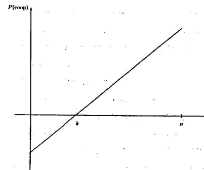
Fig. 1. Determinazione della norma di imparzialità in termini della soglia di cooperazione autosufficiente
