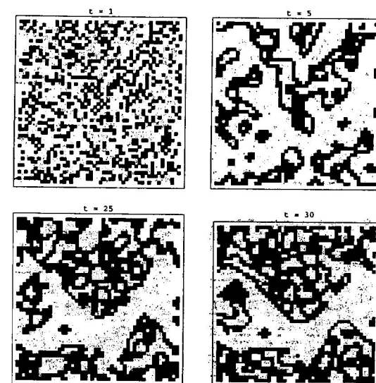
Fig. 11b. k=4 , h=7
