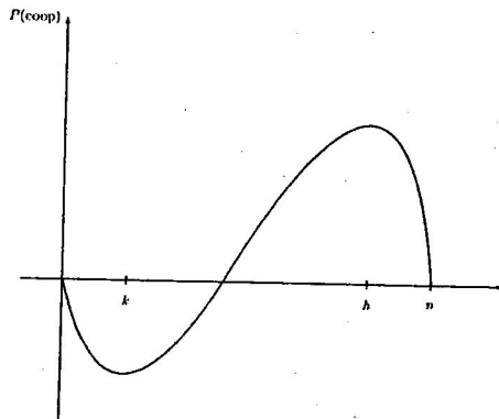
Fig. 7. Funzione nonlineare di payoff con soglia minima e massima di cooperazione per soggetti utilitaristi.
